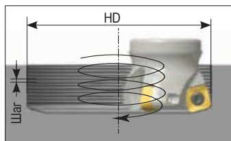
Спиральное врезание
