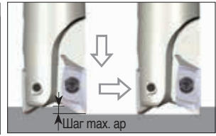
Врезание торцом
