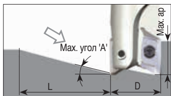
Врезание под углом
