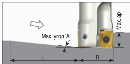
Врезание под углом
